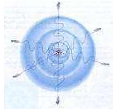
Figura 1: Onda esférica
