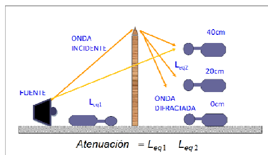
Figura 1: Esquema del sistema experimental y de la metodología de toma de datos.
