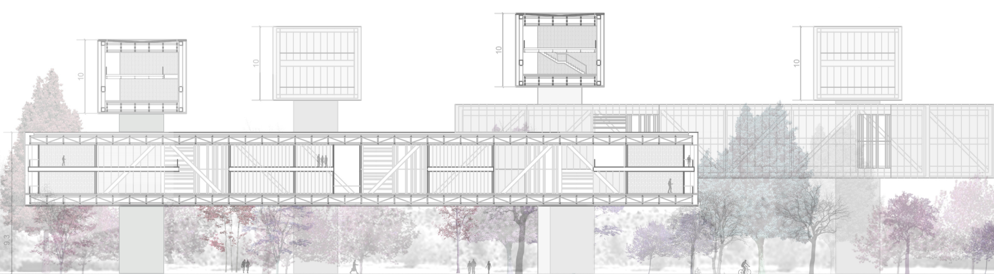
Sección B | 1:500
