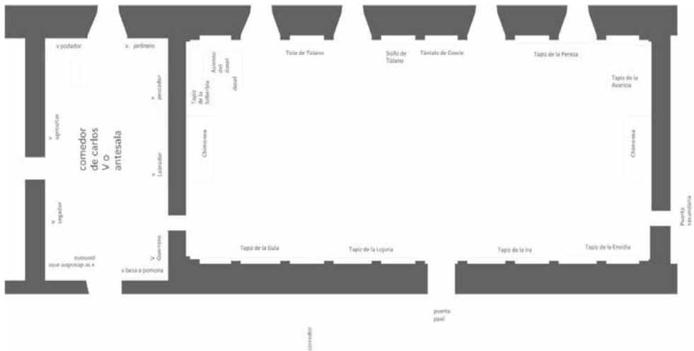
Fig. 2. Plano de la Gran Sala y de la Antecámara o comedor de Carlos V del Palacio de Binche (reconstrucción, 1549).
